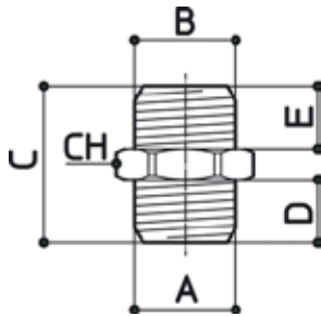
PROLUNGA CONICA TAPERED EXTENSION RALLONGE CONIQUE GERADER ÜBERGANGSTUTZEN
