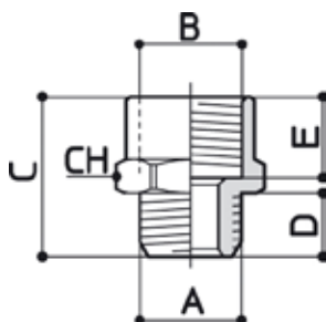
PROLUNGA CILINDRICA PARALLEL EXTENSION RALLONGE CYLINDRIQUE GERADER ÜBERGANGSTUTZEN
